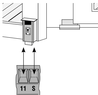
Přípojení elektrického zámku (max. 12 V – 15 W)
